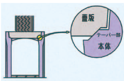
蓋掛け部イメージ ※水路幅300～600に採用(横断品除く)
